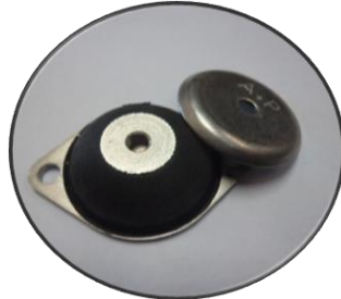
VİBRASYON TAKOZU Cihazın Teknede Monte Edildiği Yerde, Cihaz ve Tekne Arasına Konur. Böylece Cihazın Sesi ve Titreşimi Teknede Hiçbir Yere Ulaşmaz.
